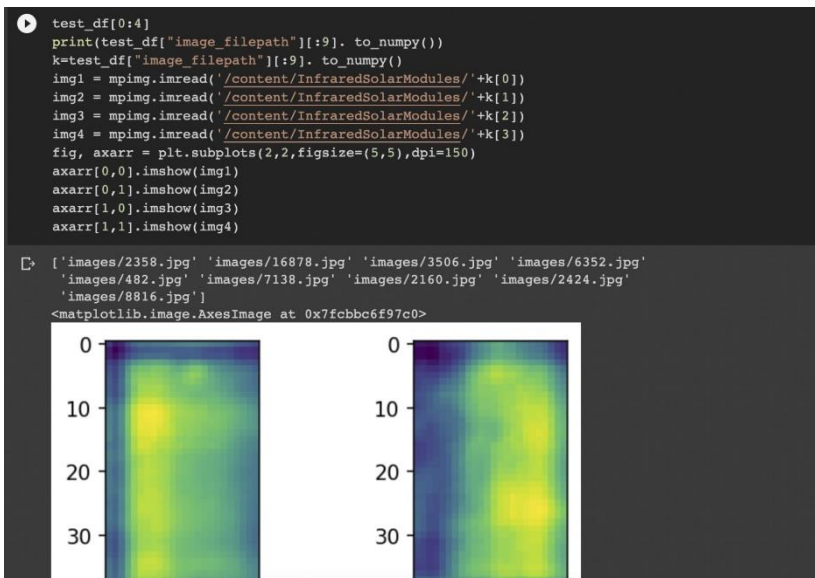
Fig. 4. Input Image
